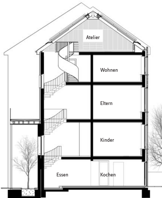
Längsschnitt | Longitudinal section
